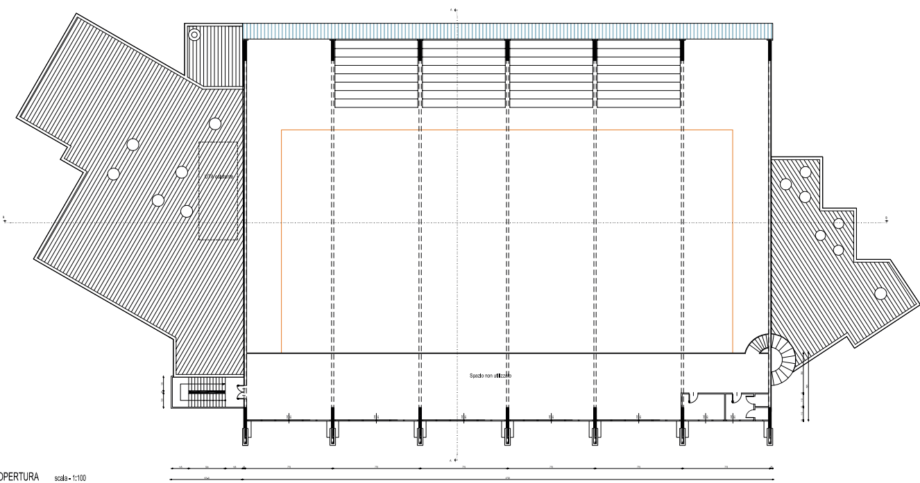
PIANTA PIANO PRIMO E COPERTURA scala - 1:100
